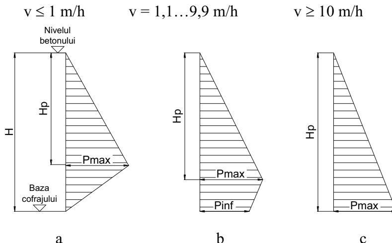
Figura C1. Distribuția presiunilor laterale, determinate de betonul proaspăt, pe pereții cofrajelor
